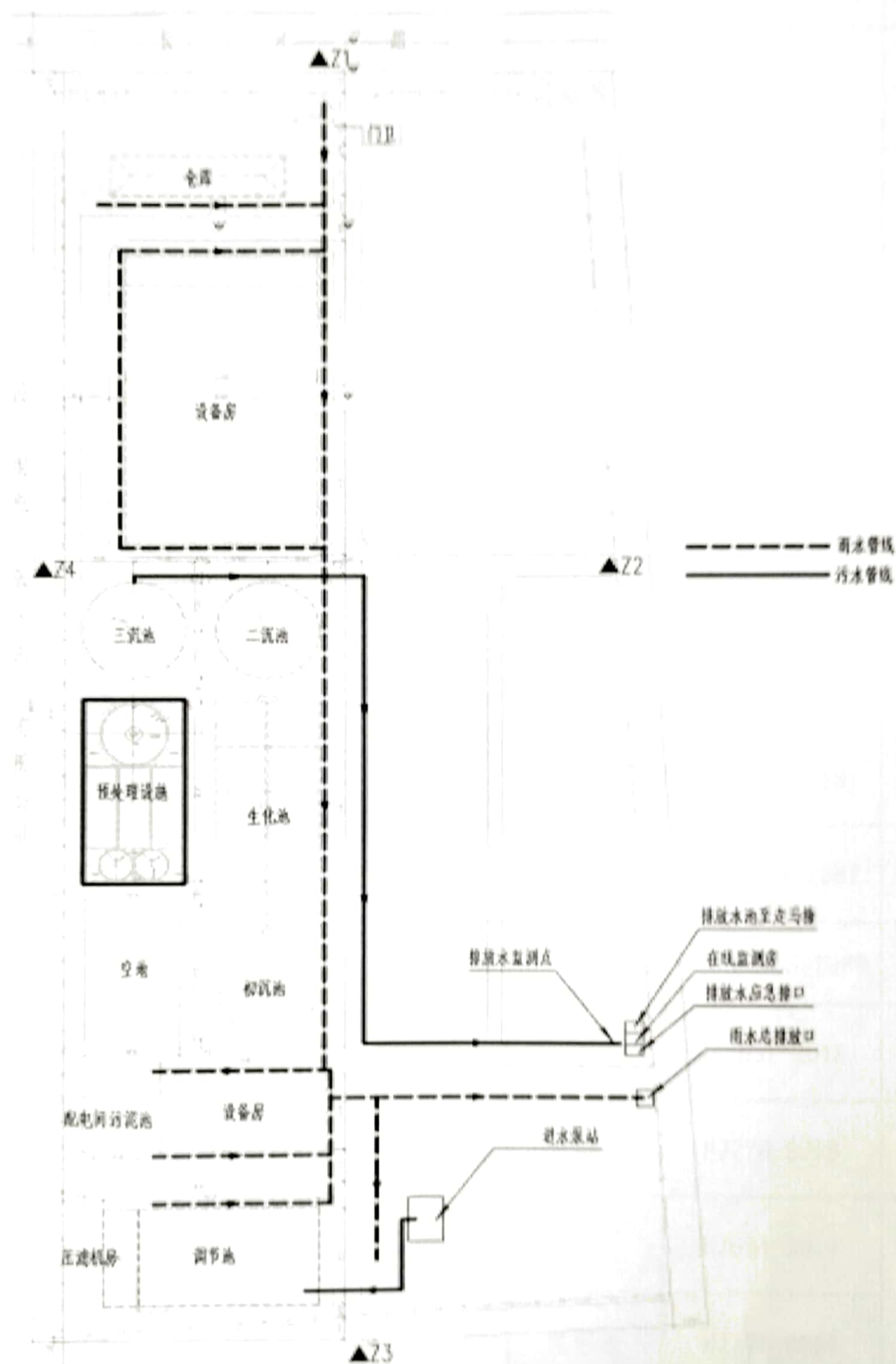
总平面布置图
