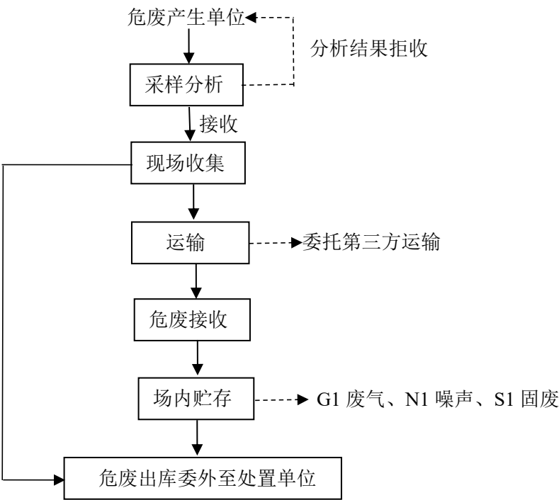
图 2-4 危废收集贮存运营流程及产污环节流程图
