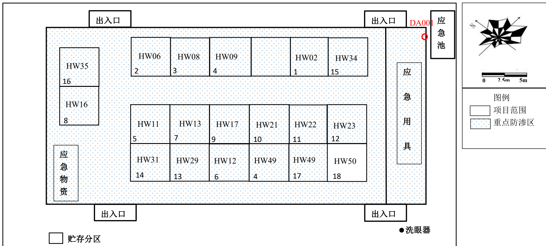
附图 10 建设项目厂区分区防渗图
